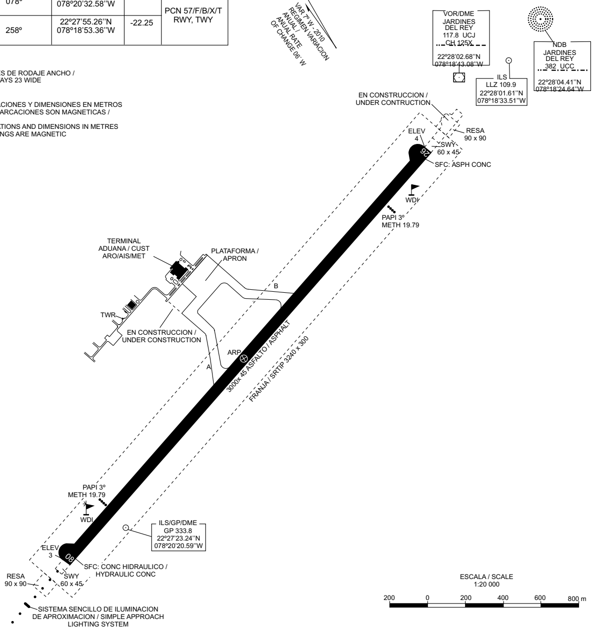
SEÑALES Y AYUDAS LUMINOSAS RWY 08/26 Y CALLES DE RODAJE DE SALIDA / MARKING AND LIGHTING AIDS RWY 08/26 AND EXIT TAXIWAYS
