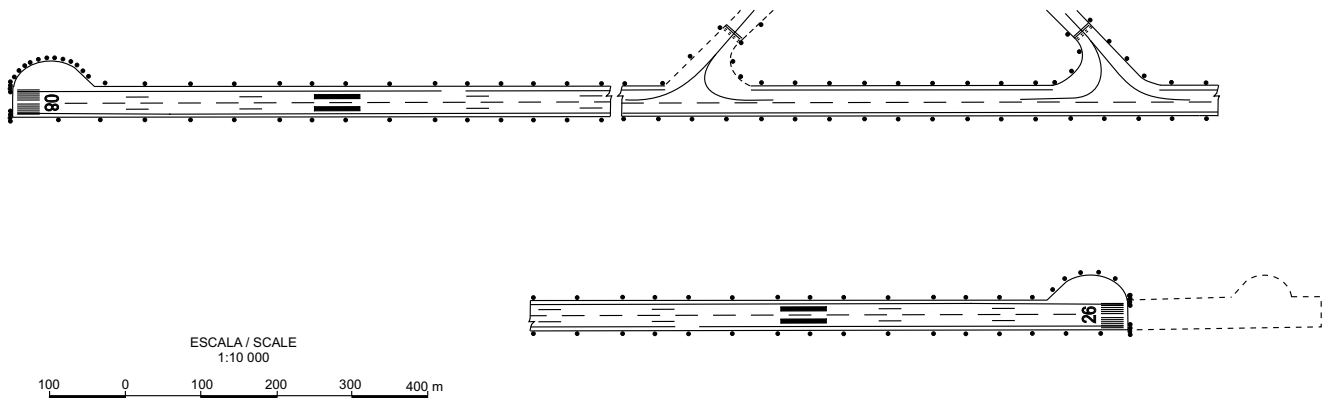
SEÑALES Y AYUDAS LUMINOSAS RWY 08/26 Y CALLES DE RODAJE DE SALIDA / MARKING AND LIGHTING AIDS RWY 08/26 AND EXIT TAXIWAYS
