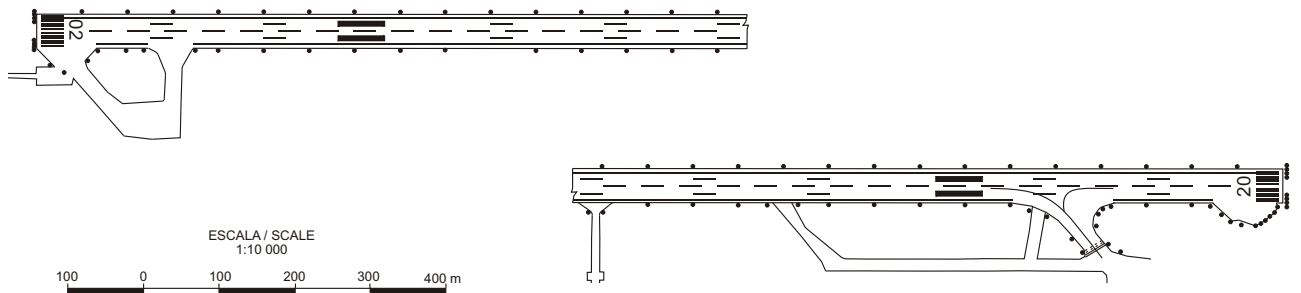
SEÑALES Y AYUDAS LUMINOSAS RWY 02/20 Y CALLES DE RODAJE DE SALIDA / MARKING AND LIGHTING AIDS RWY 02/20 AND EXIT TAXIWAYS
