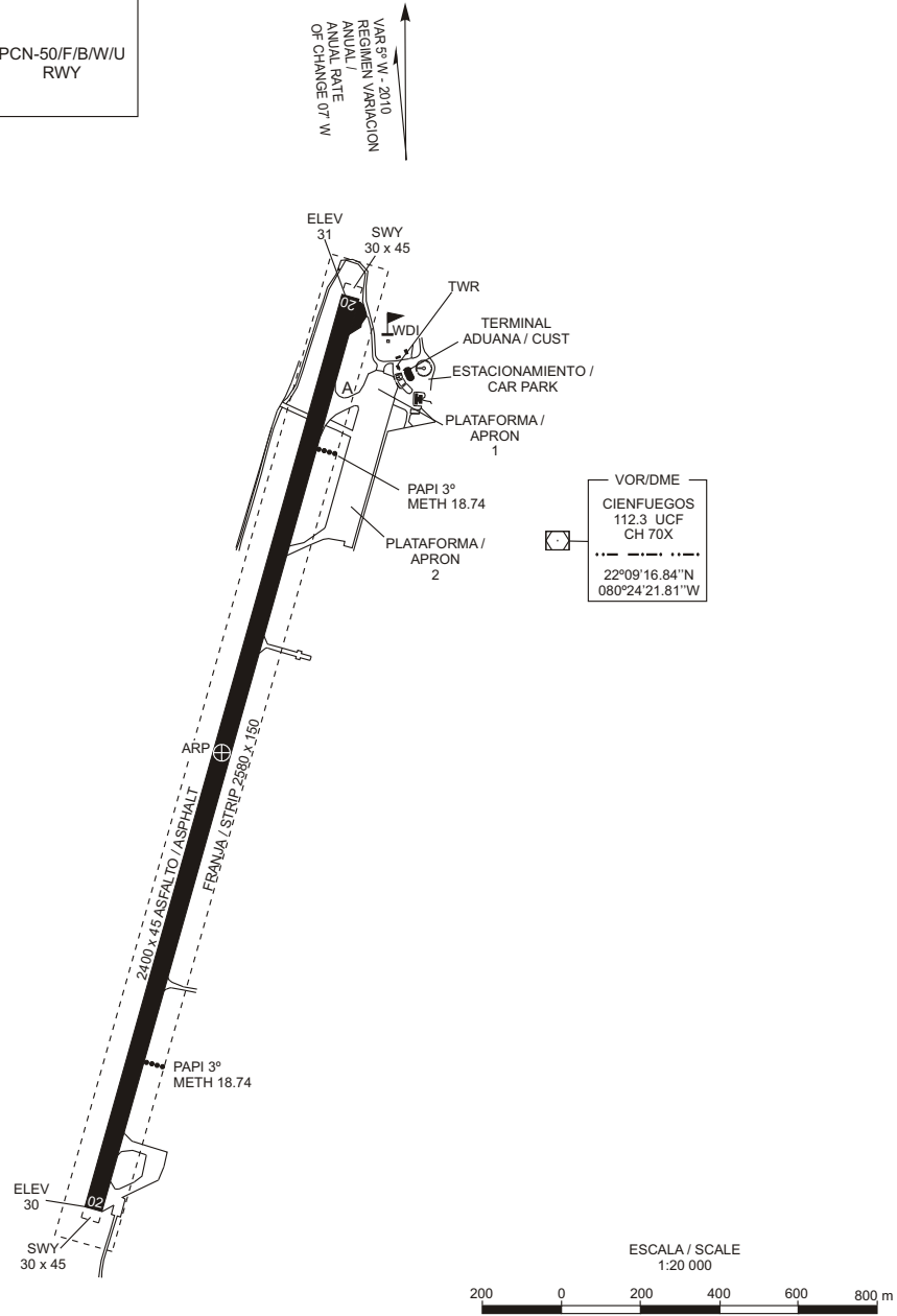
SEÑALES Y AYUDAS LUMINOSAS RWY 02/20 Y CALLES DE RODAJE DE SALIDA / MARKING AND LIGHTING AIDS RWY 02/20 AND EXIT TAXIWAYS
