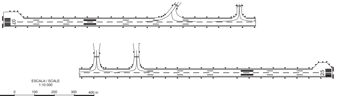
SEÑALES Y AYUDAS LUMINOSAS RWY 07/25 Y CALLES DE RODAJE DE SALIDA / MARKING AND LIGHTING AIDS RWY 07/25 AND EXIT TAXIWAYS
