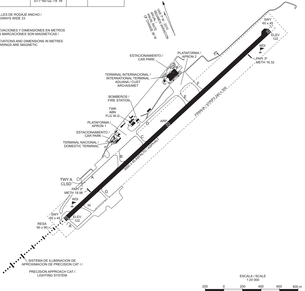
SEÑALES Y AYUDAS LUMINOSAS RWY 07/25 Y CALLES DE RODAJE DE SALIDA / MARKING AND LIGHTING AIDS RWY 07/25 AND EXIT TAXIWAYS
