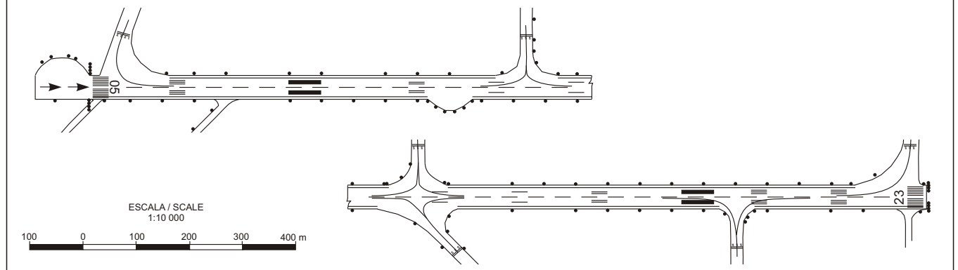
SEÑALES Y AYUDAS LUMINOSAS RWY 05/23 Y CALLES DE RODAJE DE SALIDA / MARKING AND LIGHTING AIDS RWY 05/23 AND EXIT TAXIWAYS
