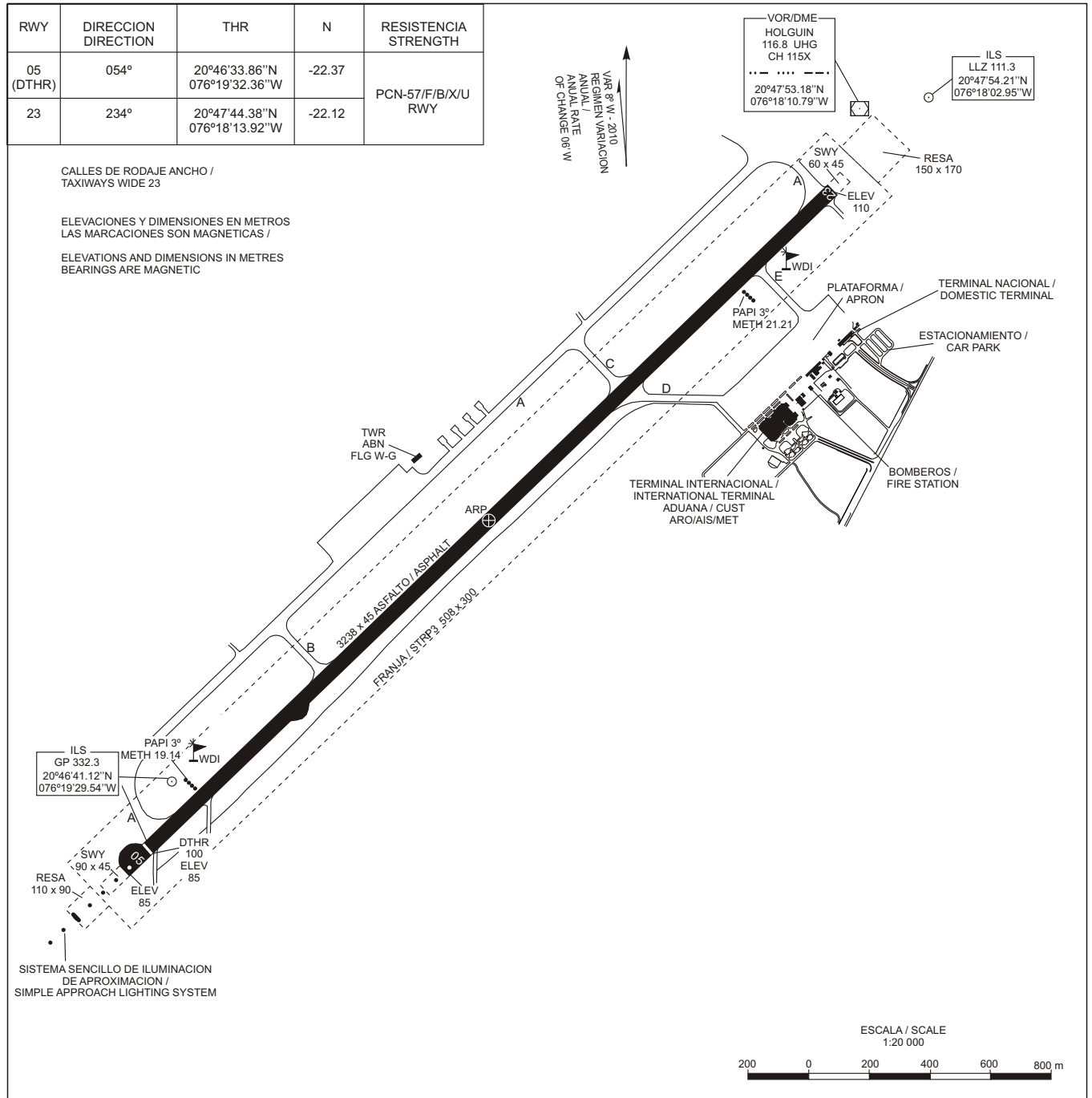
SEÑALES Y AYUDAS LUMINOSAS RWY 05/23 Y CALLES DE RODAJE DE SALIDA / MARKING AND LIGHTING AIDS RWY 05/23 AND EXIT TAXIWAYS
